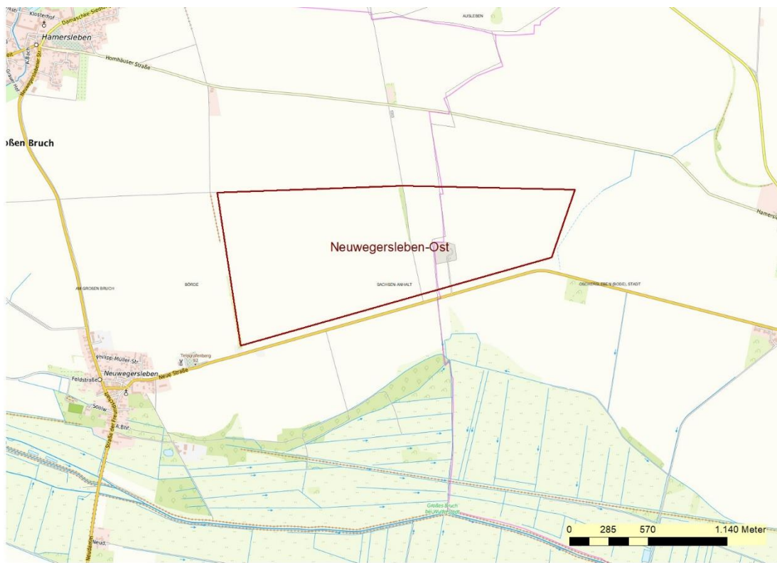
Topografische Karte, Projektion des Bergwerksfeldes Neuwegersleben-Ost
